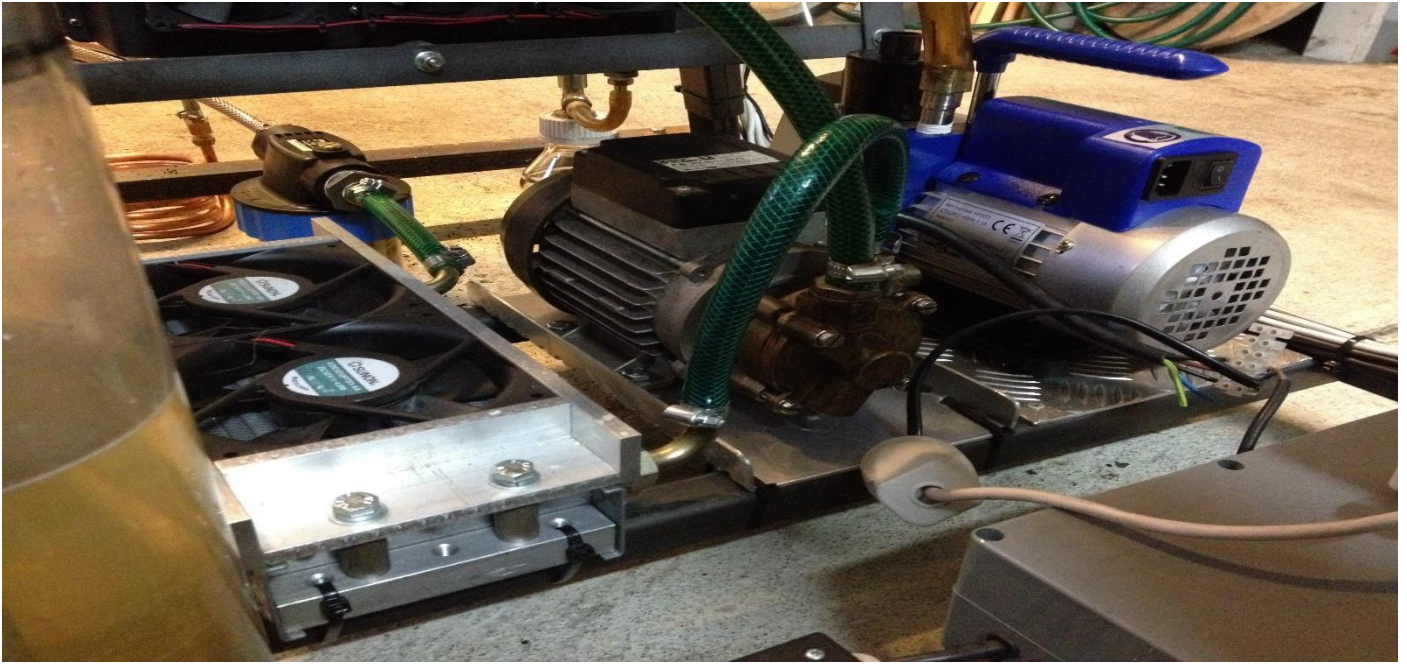
Cisterne med vaskevand + div. pumper, køler og for-filter.
